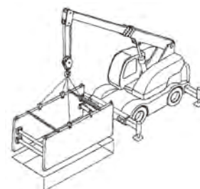
縦ばりプレートの建て込み
